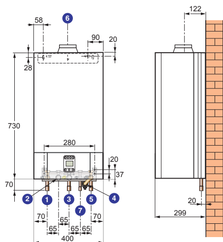
MS 24 MI MS 24 MI VMC
