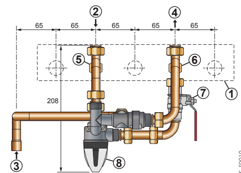
Kit de raccord. hydraulique sur un circuit solaire avec vanne directionnelle thermostatique - Colis HX 23 - (pour MS 24 MI (FF, VMC) uniqt)
